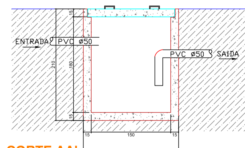
CORTE AA'
